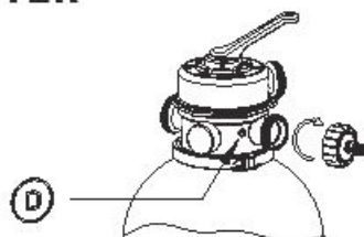
2. Schroef de tuinslangadapter (21) op poort D van de zandfilter.
