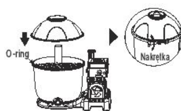
3. Upewnij się, że O-ring znajduje się na miejscu na obręczy Zbiornika Dolnego, upewnij się, że O-ring oraz obręcz Zbiornika Dolnego są czyste i wolne od szczyrbów, zadziórów, strzępów oraz piasku. Przymocuj Pojemnik Górny do Pojemnika Dolnego, załóż Kołnierz Zacisku dookoła ich połączenia i obróć nakrętkę zgodnie z ruchem wskazówek zegara, aby ją przymocować.
