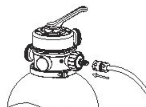
3. Bevestig de tuinslang op de tuinslangadapter(21).
