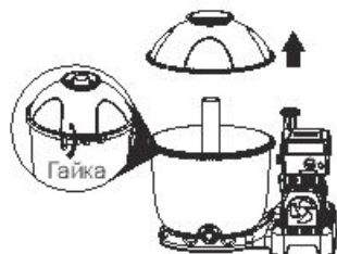
1. Поверните гайку против часовой стрелки, чтобы ослабить фланцевое крепление и снимите верхнюю часть корпуса.
