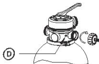
2. Навинтите переходник (21) для садового шланга на канал D песочного фильтра.
