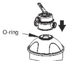
4. Podłącz Zawór Sterowania do Zbiornika Górnego, upewniając się, że O-ring znajduje się na miejscu, na obręczy Zbiornika Górnego, upewnij się, że O-ring oraz obręcz Zbiornika Górnego są czyste i wolne od szczyrbów, zadziórów, strzępów oraz piasku oraz, że rura pionowa Środkowa jest wsunięta do podstawy Zaworu Sterowania.
