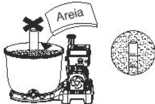
2. Adicione lentamente a areia para que o peso da areia não danifique o Skimmer, até que esta alcance um ponto entre as marcações "MÁX" E "MÍN". Não verta a areia no tubo do Cubo Colector. #20 Areia de sílica 0.45-0.85mm, aproximadamente 25 kg.
