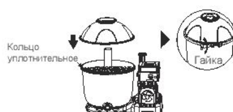
3. Убедитесь в том, что уплотнительное кольцо правильно расположено на кромке нижнего бака, а также, что кольцо и кромка чистые, без зазубрин, разрывов, мусора или песка. Соедините верхнюю и нижнюю части корпуса, наложите на место стыка хомут и закрутите гайку по часовой стрелке.
