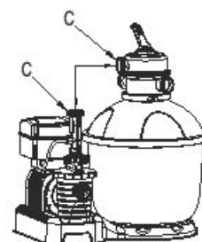
6. Bevestig de leiding op poort C van de pomp en op poort C van de regelklep, schroef de sluitringen op hun plaats. Controleer of de afdichtingen goed op beide uiteinden van de leiding zijn geplaatst.
