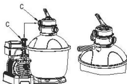
5. Что «патрубок C» на управляющем клапане совмещен с патрубком C на насосе. Поставить верхний хомут и закрутить по месту.
