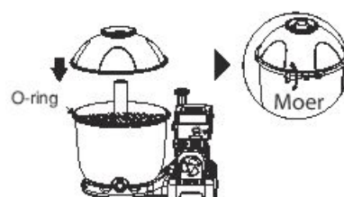
3. Zorg ervoor dat de O-ring op zijn plaats zit op de velg van de onderste tank, zorg dat de O-ring en de velg van de onderste tank schoon zijn zonder inkepingen, scheuren, krassen of zand. Maak de bovenste tank vast aan de onderste tank, plaats de flensklep over de naad en draai de moer rechtsom om hem vast te zetten.
