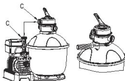
5. Controleer voor het vastmaken of poort C op de regelklep goed staat ten opzichte van poort C op de pomp. Bevestig de bovenste flensklep en schroef hem vast.
