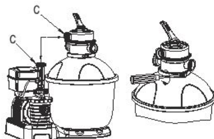
5. Należy upewnić się czy złącze C zaworu kontrolnego jest zrównane ze złączem C pompy. Załóż górny zacisk i dokręć go.
