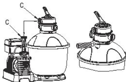
5. Certifique-se que a Porta C na válvula de controlo está alinhada à porta C na bomba. Engate o grampo do flange superior e aperte-o na posição.
