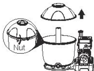
1. Gire a porca no sentido anti-horário para soltar a flange de fixação e remova o tanque superior.
