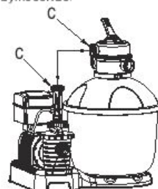
6. Podłącz rurę do złącza C pompy oraz do złącza C zaworu kontrolnego, dokręć pierścienie zaciskające. Upewnij się że uszczelka jest właściwie założona na obu końcach rury.
