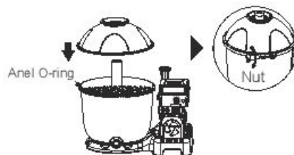
3. Certifique-se que o O-ring está no seu lugar na borda do Tanque Inferior, certifique-se que o O-ring e a borda do Tanque Inferior estão limpos sem cortes, rasgos, arranhões ou areia. Conecte o tanque superior ao tanque inferior, coloque a flange de fixação na junção e gire a porca no sentido horário para apertar.
