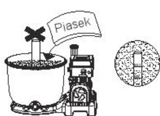
2. Powoli dodawaj piasek tak, aby waga piasku nie doprowadziła do uszkodzenia Cedzidla do momentu aż osiągnie on poziom oznaczony pomiędzy „MAX” i „MIN”. Nie wysypuj piasku do rurki Środk. # 20 piasek krzemionkowy 0,45-0,85mm, około 25 kg.
