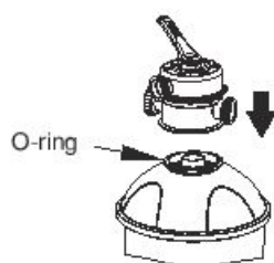
4. Bevestig de controleklep aan de bovenste tank, waarbij u ervoor zorgt dat de O-ring op zijn plaats zit op de velg van de bovenste tank. Zorg ervoor dat de O-ring en de velg van de bovenste tank schoon zijn zonder inkepingen, scheuren, krassen of zand en dat de verticale pijp van de naaf in de basis van de controleklep is gestoken.
