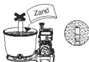
2. Voeg het zand langzaam toe zodat het gewicht van het zand de skimmer niet beschadigt, totdat het tussen de merkjes "MAX" en "MIN" reikt. Giet het zand niet in de pijp van de collectornaaf. #20 Silica zand 0.45-0.85mm, ongeveer 25 kg.
