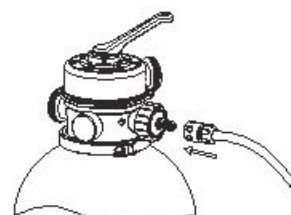
3. Подсоедините садовый шланг к переходнику (21) для садового шланга.
