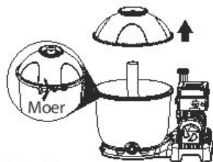
1. Draai de moer linksom om de flensklep vrij te geven en verwijder de bovenste tank.
