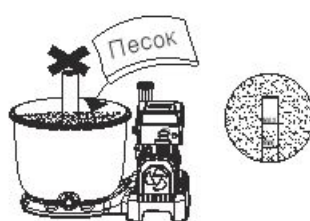
2. Медленно всыпьте песок, так чтобы его вес не повредил скиммер, пока количество песка не достигнет промежутка между отметками «МАКС.» и «МИН.». Не засыпайте песок в трубку коллекторной втулки. №20 Песок Silica, 0,45-0,85 мм, приблизительно 25 кг.
