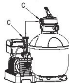
6. Engate a tubulação à porta C da bomba e à Porta C da válvula de controlo, aparafuse os anéis de bloqueio rosqueados na posição. Certifique-se que a arruela está posicionada adequadamente em ambas as extremidades da tubulação.
