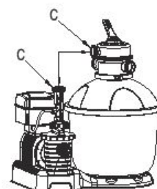
6. Соедините трубой патрубок C насоса и патрубок C управляющего клапана, закрутите резьбовые уплотнительные кольца до упора. Убедитесь в том, что шайбы правильно установлены на обоих концах трубки.
